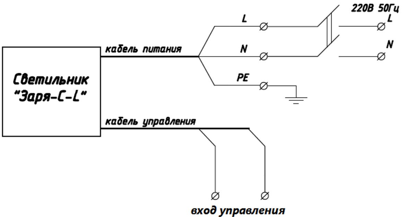
Рисунок 1.10. Схема подключения светильника «Заря-С-L» исп. «К/У», «К/П»
