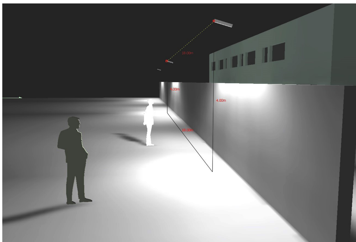
Рисунок 1.3 - Схема установки светильников, обеспечивающая освещенность на уровне земли не хуже 10 лк в полосе 3 м при неравномерности не выше 10 дБ.
