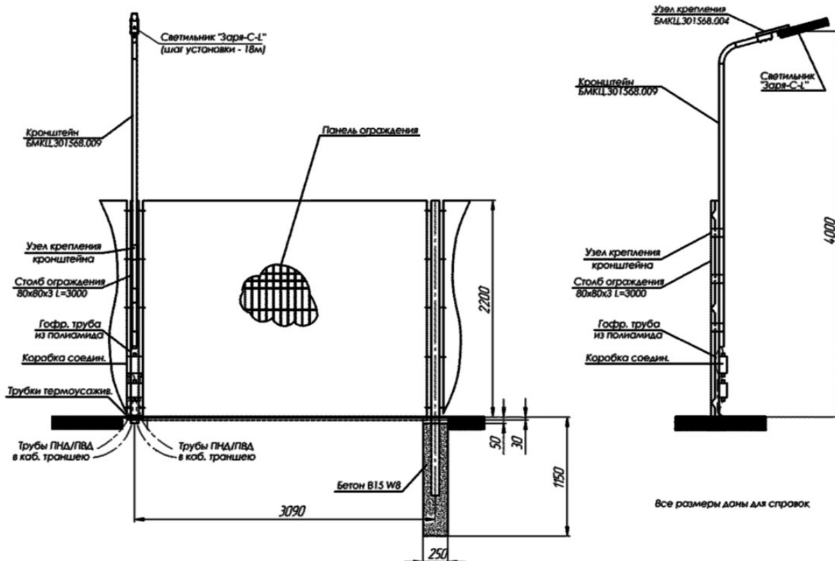
Рисунок 2.1. Монтаж светильника на сварное проволочное ограждение с опорными столбами квадратного сечения 50×50...80×80 мм (кронштейн «Заря-К-У» БМКЦ.747132.005, узел крепления «Заря-УК-4» БМКЦ.301568.004)
