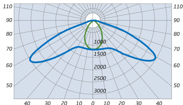
Рисунок 1.2 - Кривая силы света светильника «Заря»
