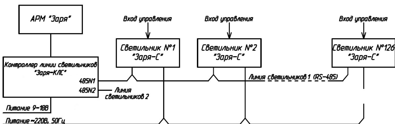
Рисунок 1.9 - Схема подключения светильников «Заря-С» к контроллеру «Заря-КЛС»
