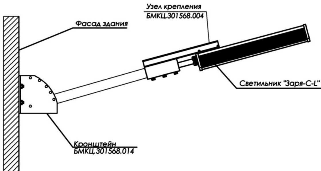
Рисунок 2.2. Установка светильника на фасад здания с помощью узла крепления БМКЦ.301568.004 и кронштейна «Заря-К-14» (БМКЦ.301568.014).
