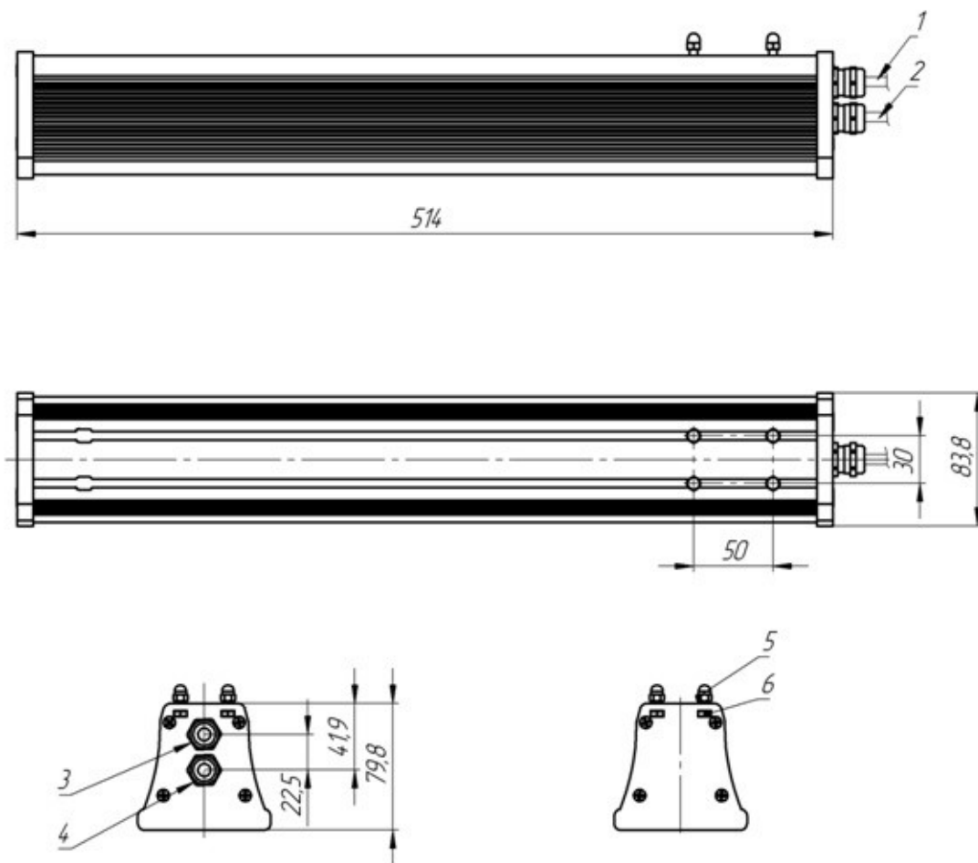
Рисунок 1.1 - Светильник «Заря-С» («Заря-С-Л»):
