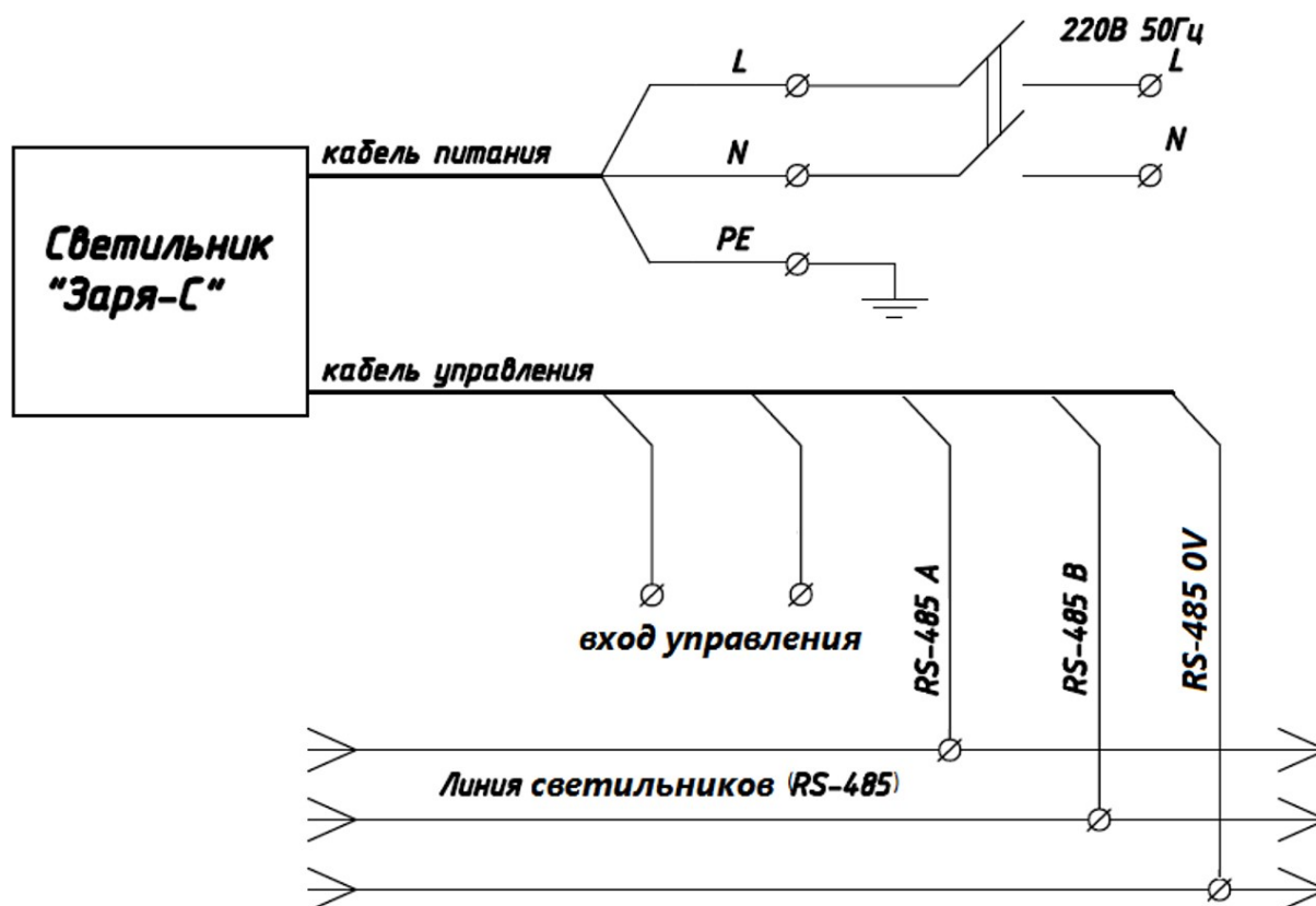
Рисунок 1.8 - Схема подключения светильника «Заря-С» к линии интерфейса RS-485.
