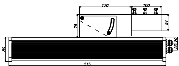
Светильник "Заря-С" Габаритный чертёж
