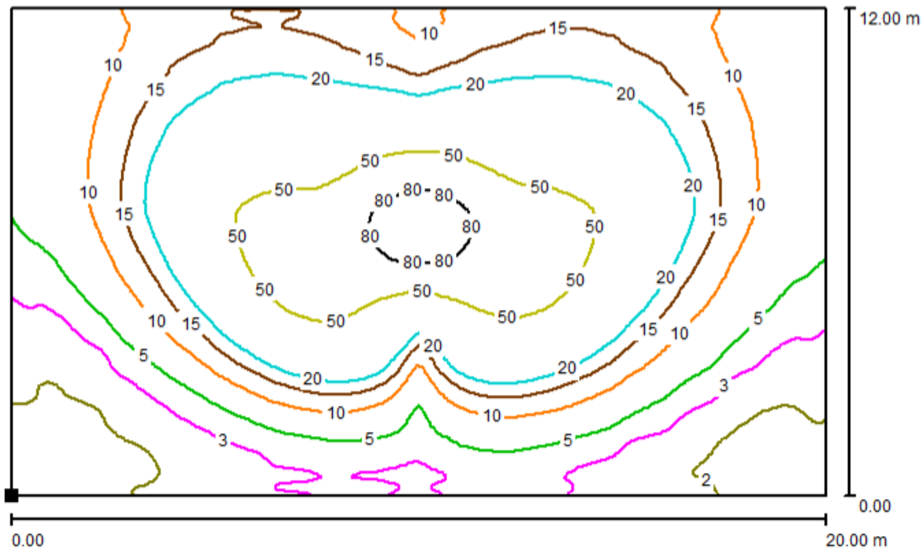
Диаграммы распределения горизонтальной освещенности (лк) на уровне земли при высоте установки одиночного светильника 4 м.
