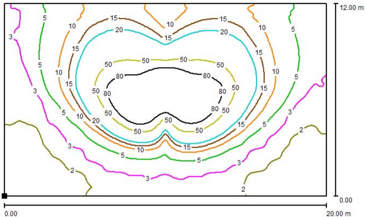
Диаграммы распределения горизонтальной освещенности (лк) на уровне земли при высоте установки одиночного светильника 3 м.
